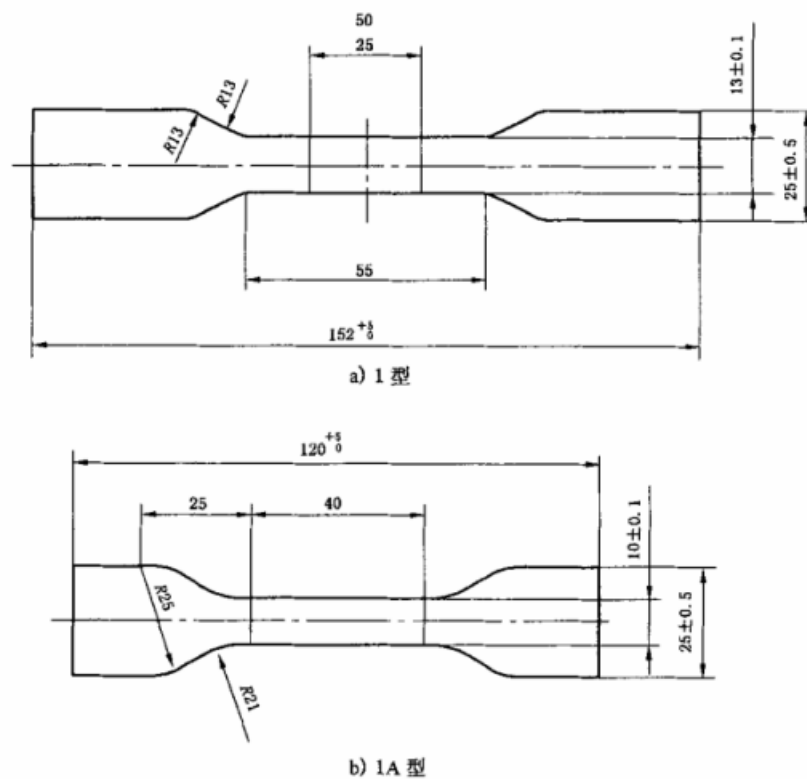
图 1 刀模尺寸示意图
