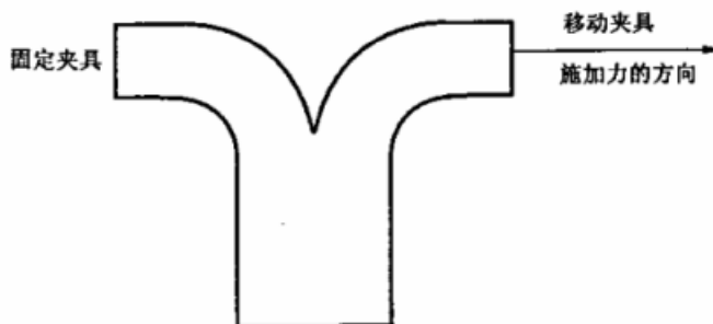
图 2 试样夹持示意图
