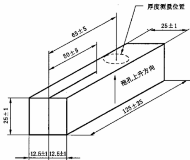
图 1 撕裂试样
